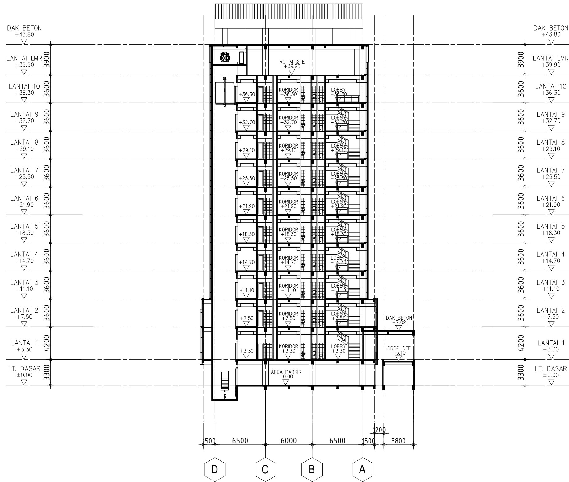
01 POTONGAN B-B SKALA 1:300
