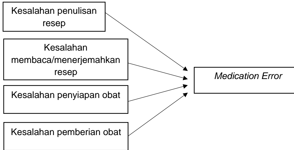
Gambar 3. Kerangka Konsep
